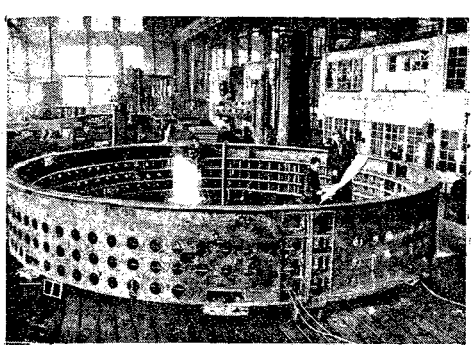
W licznych zakładach radzieckich produkują się potężne, jedyne na świecie pod względem rozmiarów i mocy instalacje elektryczne dla gigantycznych słowni wodnych na Woldze, Donie, Dnieprze i Amu Darii. Na zdjęciu budowa hydrogeneratorów dla zapory Cymlińskiej w fabryce „Elektrosila” w Leningradzie. Foto CAF.
