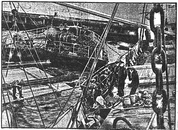
WYCIĄGANIE OKRĘTU, ZATOPIONEGO U WJAZDU DO PORTU GDYNSKIEGO. Wyciągnięcie dalszego z pośród wielu zatopionych okrętów polskich zostało dokonane. Polski parowiec „Toruń” zamykał jeden z wjazdów do portu gdyńskiego. Tylko komin i nadbudówki pokładowe były nad wodą. Aby móc wypompować wodę, na przednim otworze ułożona została drewniana platforma, obciążona żelazem. Praca nad ostatecznym wyciągnięciem okrętu pójdzie szybciej i okręt wydobyty zostanie na powierzchnię.
