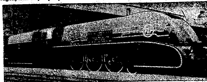
Pierwsza polska lokomotywa aerodynamiczna. Zdjęcie nasze przedstawia pierwszą polską lokomotywę aerodynamiczną, wykonaną przez Fabrykę Lokomotyw w Chranowcu. Lokomotywa ta, przeznaczona dla Działu Polskiego na Wystawie Światowej w Paryżu, może rozwijać szybkość 140 km. na godz.
