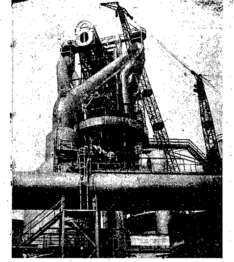
12. bm. został oddany do użytku wielki piec „B” w hucie „Kościuszk”. W uroczystym uruchomieniu pieca wzięli udział premier Józef Cyrankiewicz.
