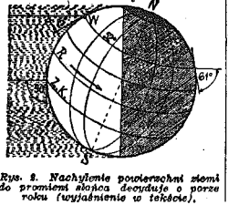
Fig. 2. Nachylenie powierzchni ziemi do promieni słonecznych...
