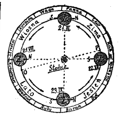
Fig. 1. Pory roku są spowodowane obrotem ziemskim...
