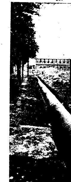
W pogłębianiu pracowni prowadzonych jest budowa szwedzkiej wodociągowej sieci w Sosnowcu. Koszt tych robót wyniesie ponad 20 milionów zł. Z rurociągu tego korzystają będą także wszystkie osiedla fabryczne.
