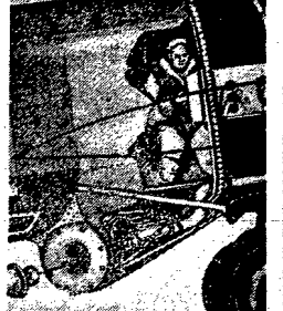
Wylot rury wlewniej zbiornika. Widoczny jest też przycięany zawór powietrznego-przewodu-benzynowego.
