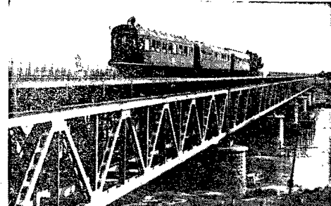
Dwa lata trwały intensywne prace przy odbudowie zniszczonego przez Niemców mostu kolejowego pod Cytadela. Dziś stanowi on najważniejszą część wielkiej arterii kolejowej, łączącej wschodnie polacie kraju z resztą Polski. Patrząc na stalowe kratownice mostu, wsparcie na kamiennych i betonowych filarach, nie przyjdzie nam na myśl, że trzy lata temu filary leżały w gruzach, a przeszła na dnie rzeki.
