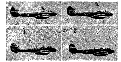
Wyrzucenie pilota sposobem automatycznym wraz z fotelom; w stadium końcowym następuje otwarcie spadochronu. Samolot „Gloster Meteor” robi 720 km. na godzinę.
