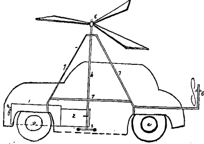
Tak wygląda auto-pter, samochód latający, według opatentowanego w Szkocji wynalazku polskiego: 1) silnik z kompresorem, 2) skrzynka biegów, 3) łożysko, 4) os napędowa rotora (wiatrak), 5) rotor, 6) śmigło pomocnicze, 7) płaszczyzna składowania.
