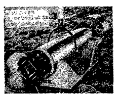
„Ptak”, czyli magnetometr napowietrzny. Zajęty kapłur przedni, pod którym widoczna jest skomplikowany mechanizm, „odczuwający” zmiany magnetyczne, powiązane z takim czy innym układem warstwic skalnych.
