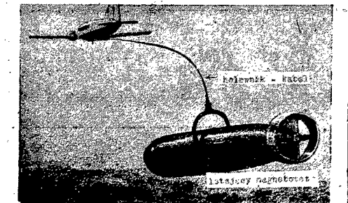
Magnetometr napowietrzny „ptak” holowany jest za samolotem i notuje zmiany magnetyczne pola, dając w ten sposób geofizykom informacje nie tylko o rodzaju pokładów górnictwa, lecz także o grubości poszczególnych złóż.
