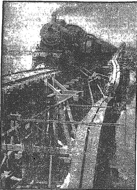
W krótkim czasie po wysadzeniu mostu przez cofających się Francuzów oddziały saperów przystąpiły do odbudowy. Na zdjęciu próba obciążenia prowizorycznego mostu
