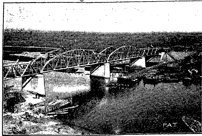
Nowy most drogowy na Polesiu. Podajemy fotografie świeżo otwartego mostu drogowego przez rzekę Pinę. Most ten zbudowany na terenie bagnistym (na 133 m. długości) i stanowi piękny okaz polskiego budownictwa mostowego.
